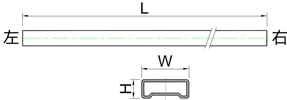
图 22 SOP&TSSOP 料管包装图
