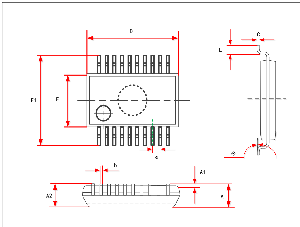
图 15 SOP20 封装图
