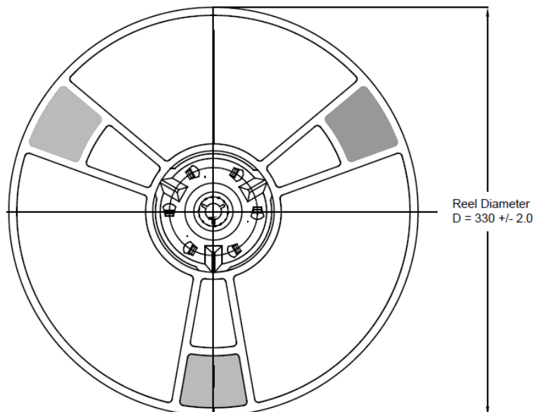
图 19 卷盘尺寸
