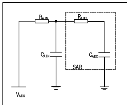
图 12 ADC 的典型应用
