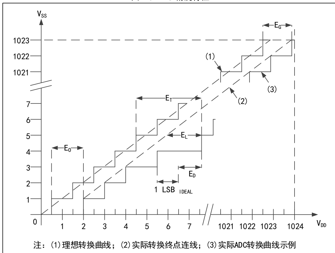
图 13 ADC 精度特性
