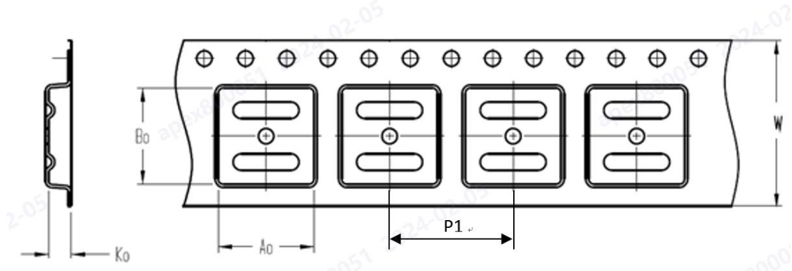
图 17 带状包装规格图
