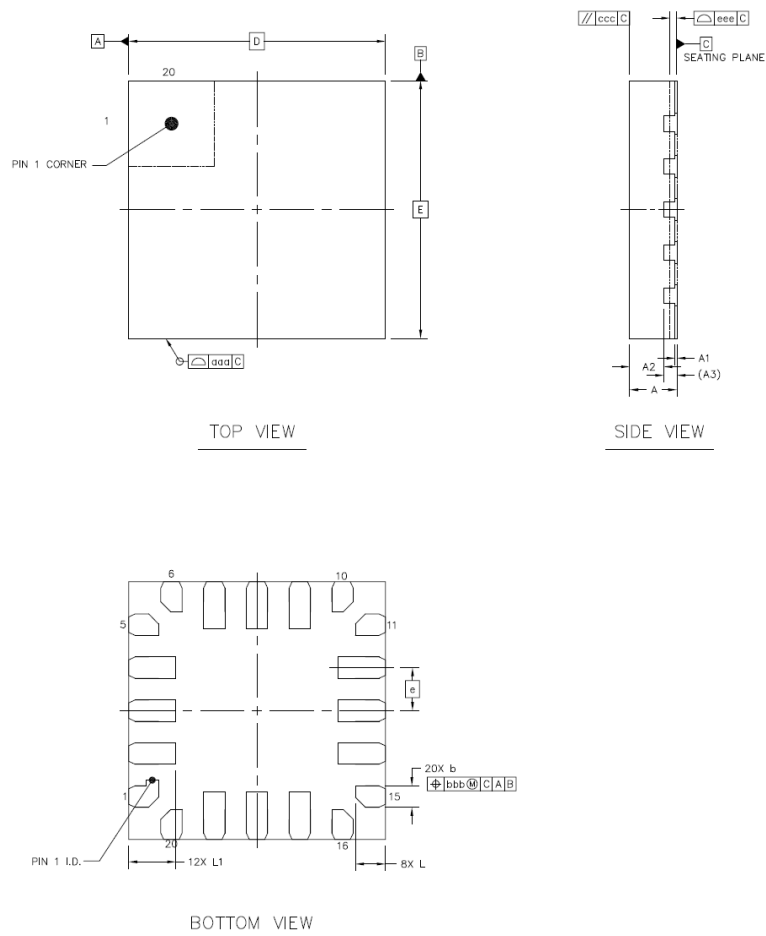
图 16 QFN20 封装图
