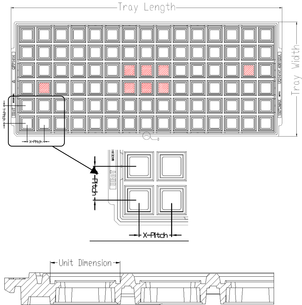
图 21 纸盘尺寸
