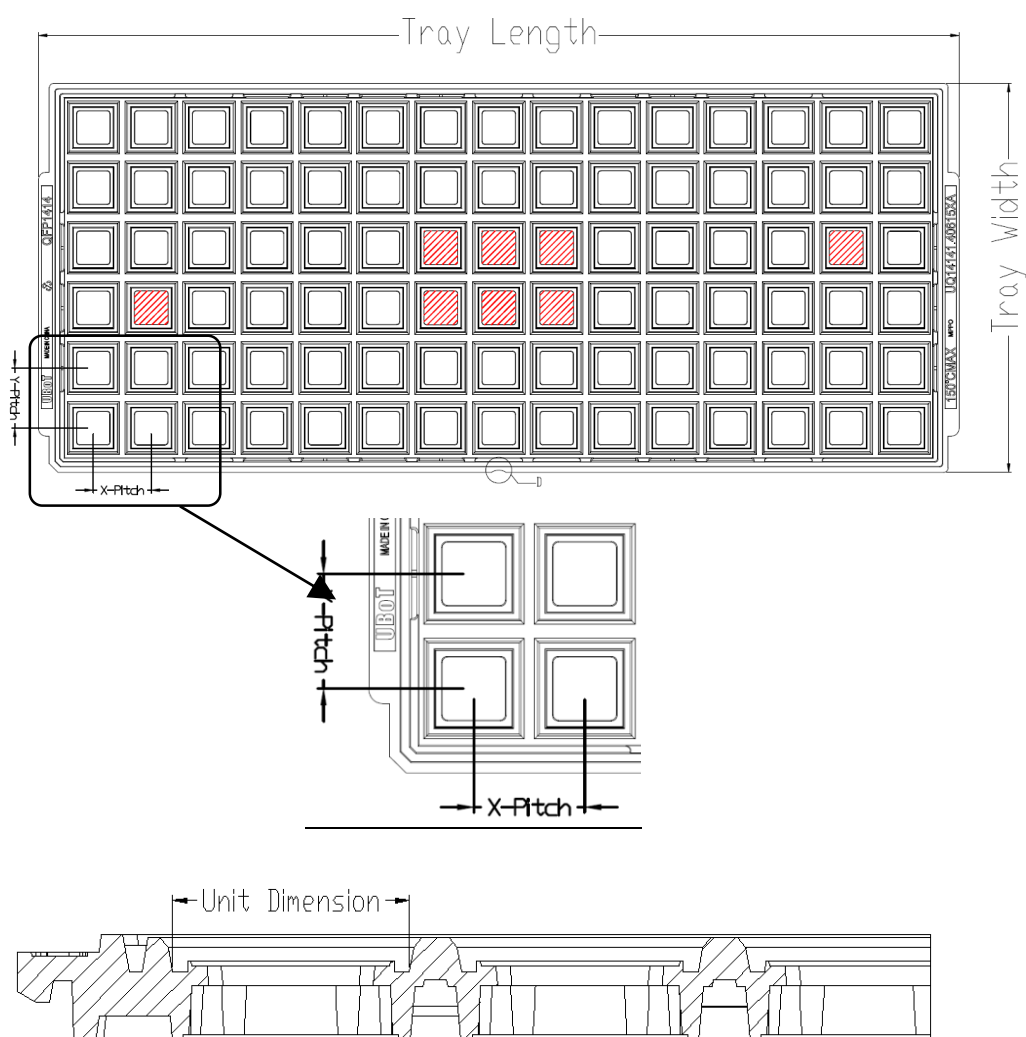
图 23 纸盘尺寸
