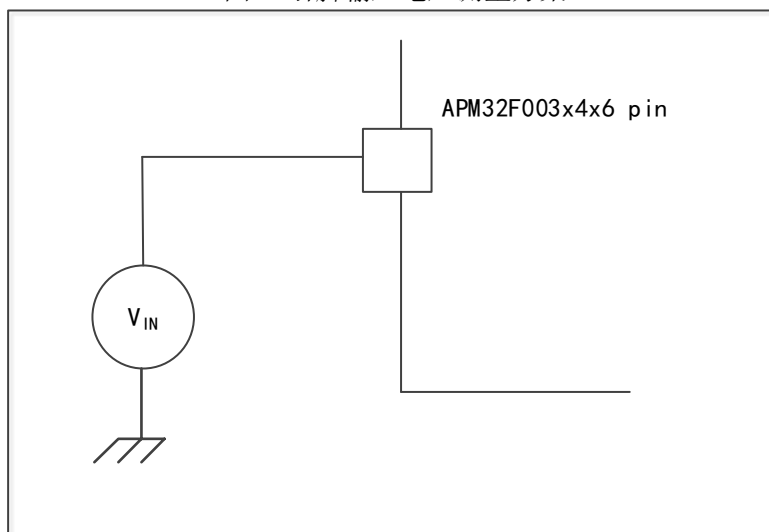
图 8 引脚输入电压测量方案
