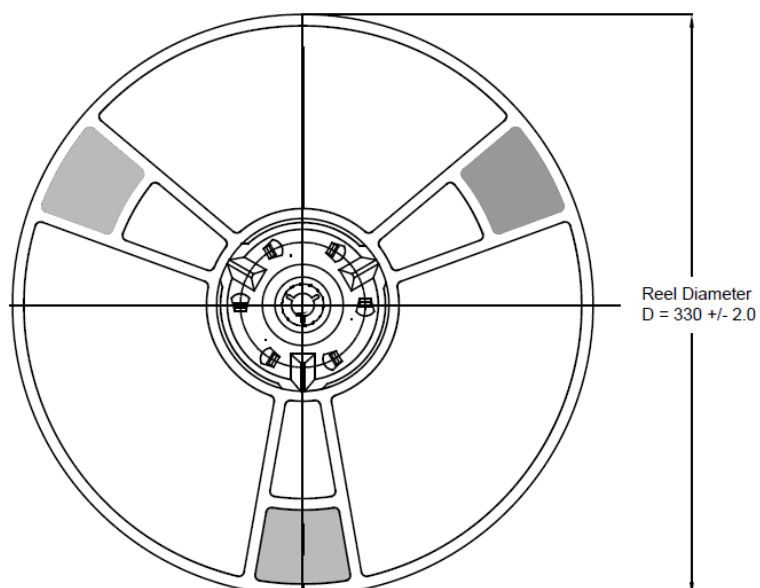
图 21 卷盘尺寸
