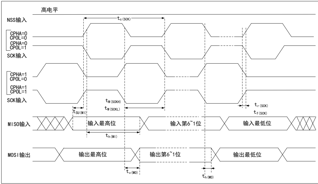
图 12 SPI 时序图—主模式(1)
