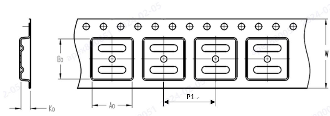
图 19 带状包装规格图
