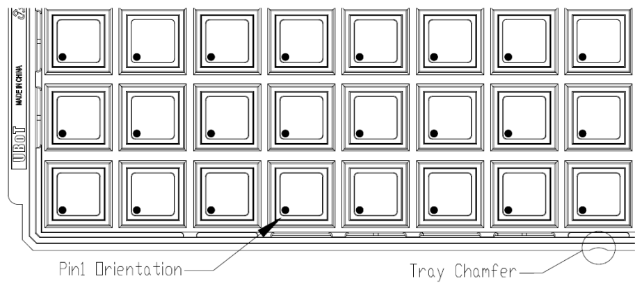
图 22 托盘包装示意图
