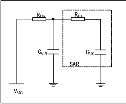
图 13 ADC 的典型应用
