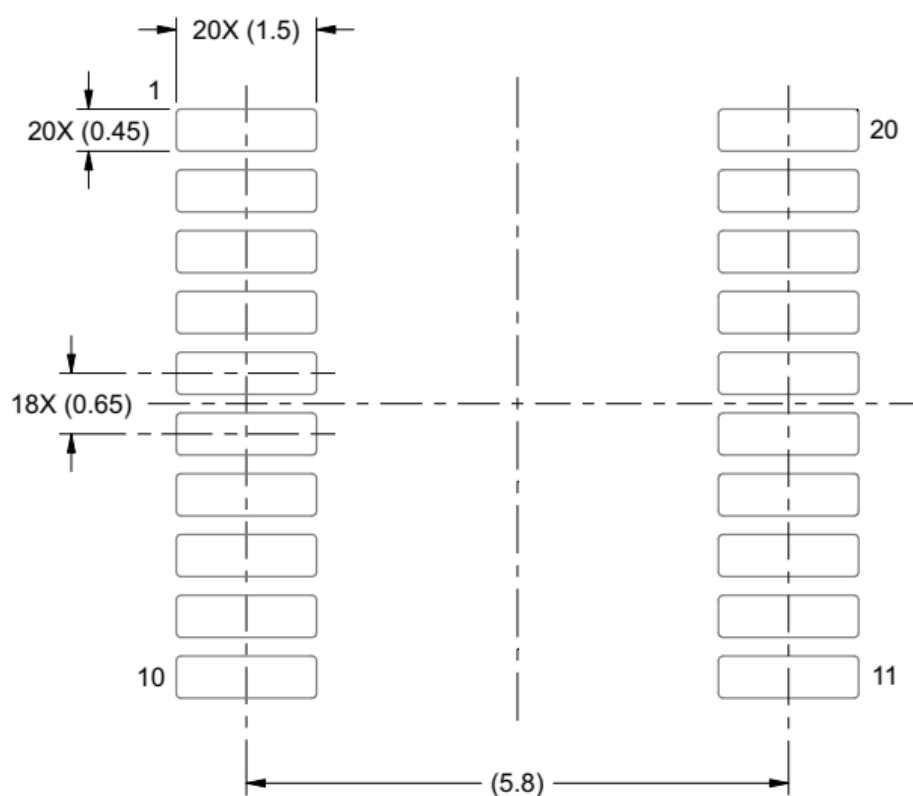
图 16 TSSOP20 焊接 Layout 建议
