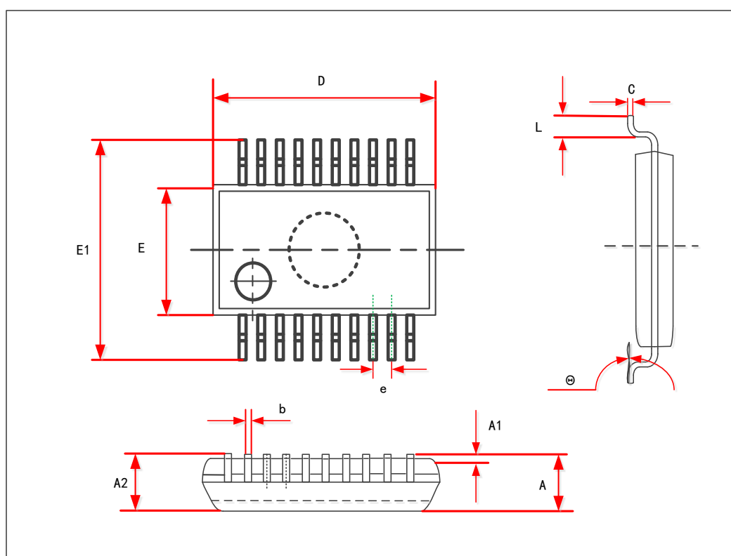
图 17 SOP20 封装图
