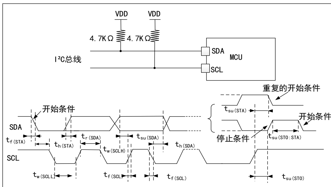
图 9 总线交流波形和测试电路
