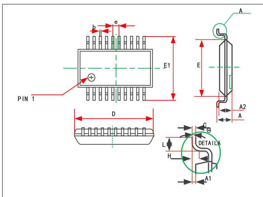
图 15 TSSOP20 封装图
