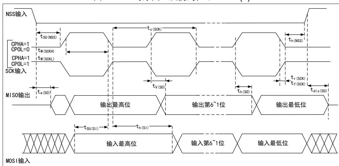
图 11 SPI 时序图—从模式和 CPHA=1(1)
