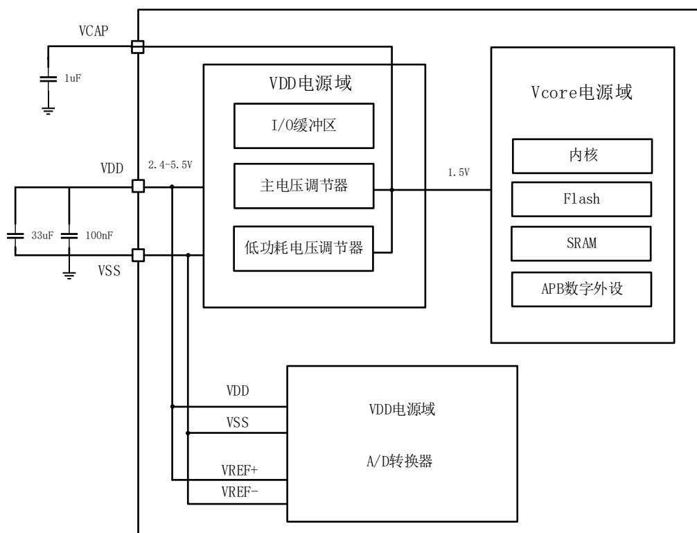
图 6 电源方案
