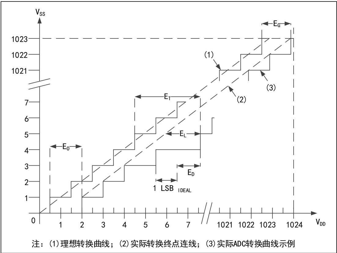
图 14 ADC 精度特性
