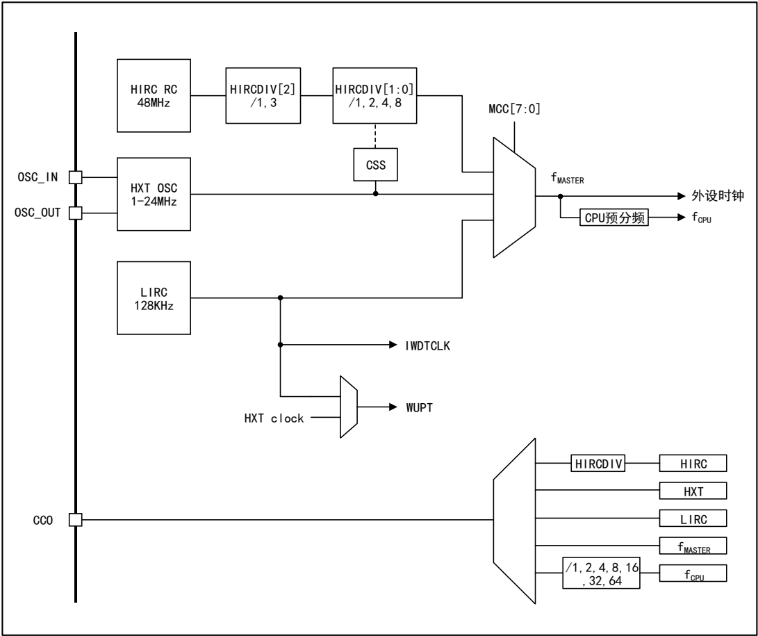
图 5 APM32F003x4x6 系列时钟树
