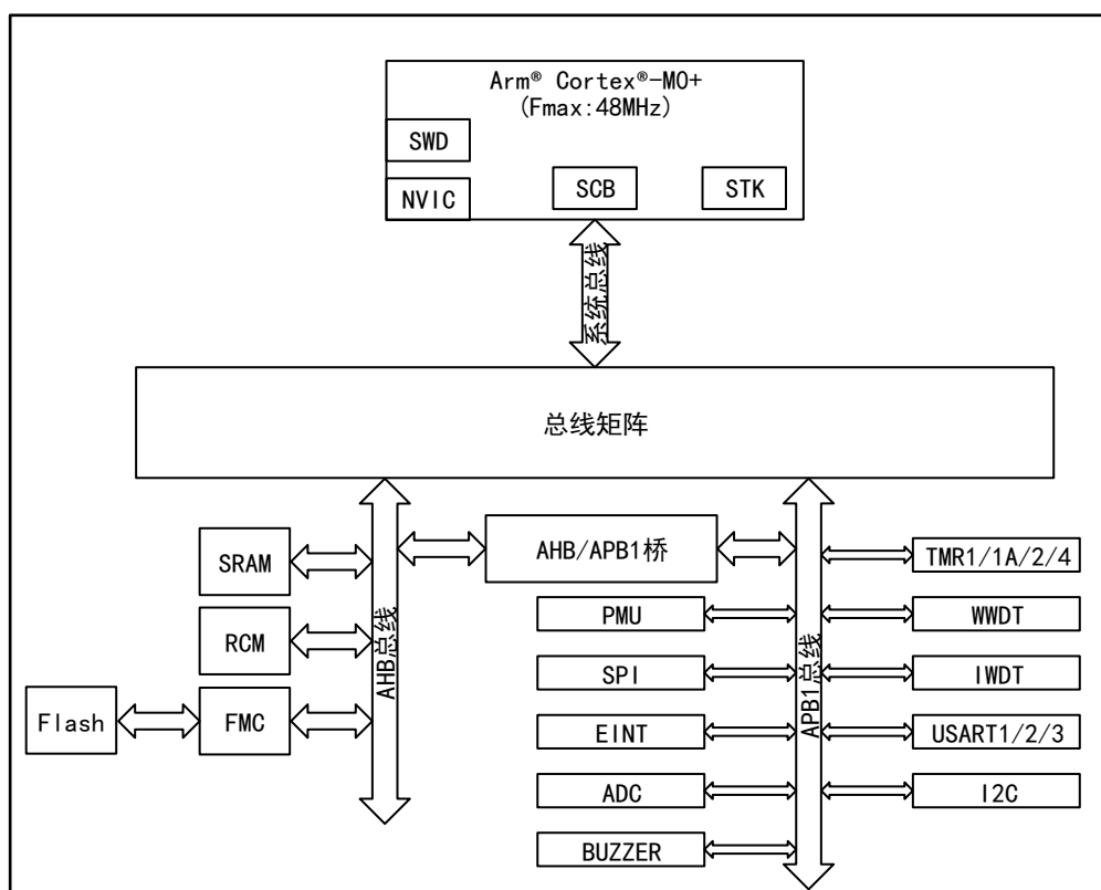
图 3 APM32F003x4x6 系列系统框图
