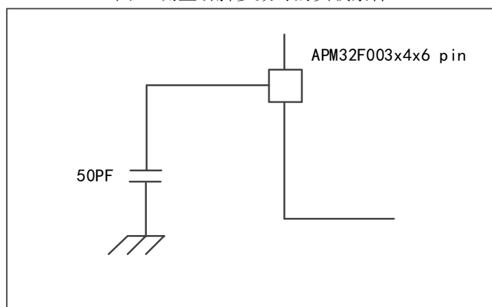
图 7 测量引脚参数时的负载条件
