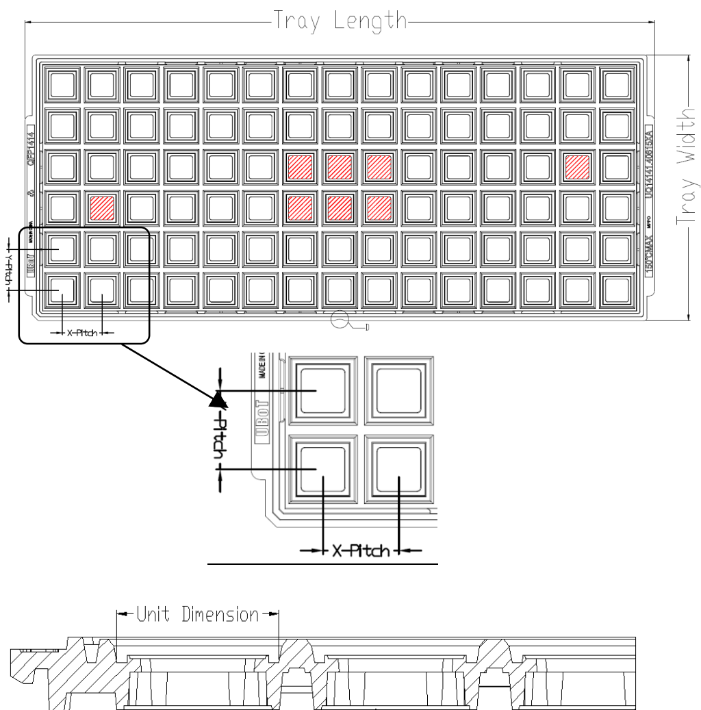
图 23 纸盘尺寸
