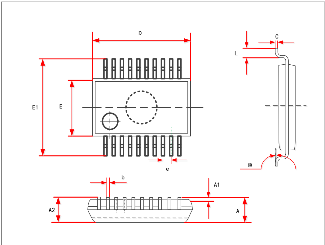
图 17 SOP20 封装图
