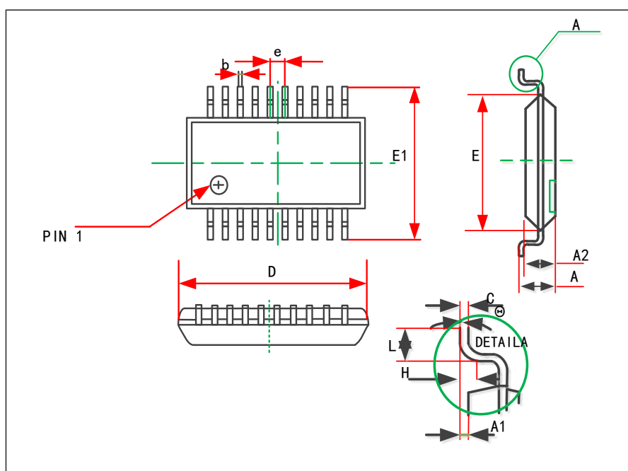
图 15 TSSOP20 封装图
