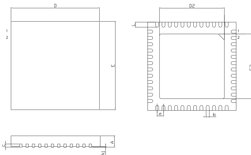
图26 QFN48 封装图
