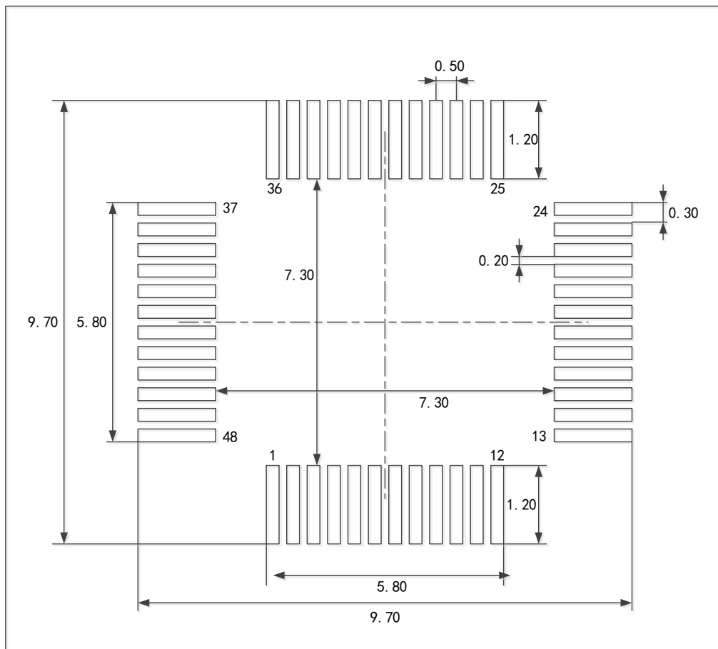
图21 LQFP48 焊接 Layout 建议
