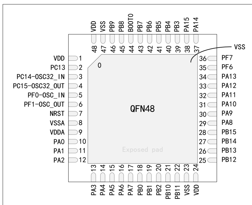
图7 APM32F030x6x8 系列 QFN48 引脚配置图
