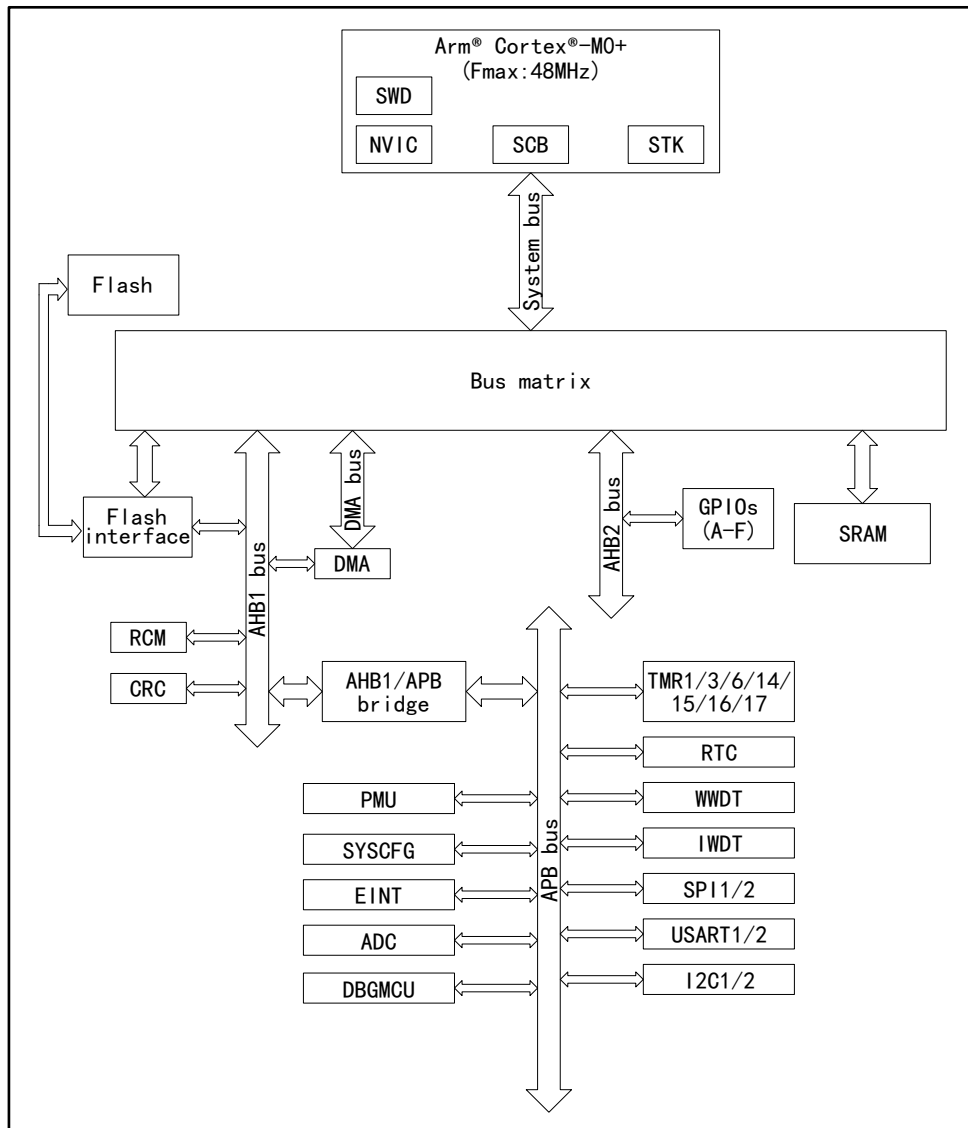
图1 系统框图
