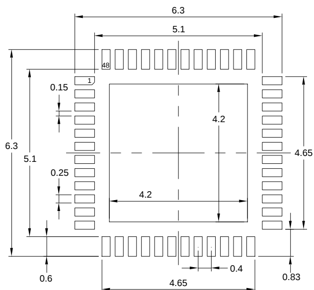
图27 QFN48 焊接 Layout 建议
