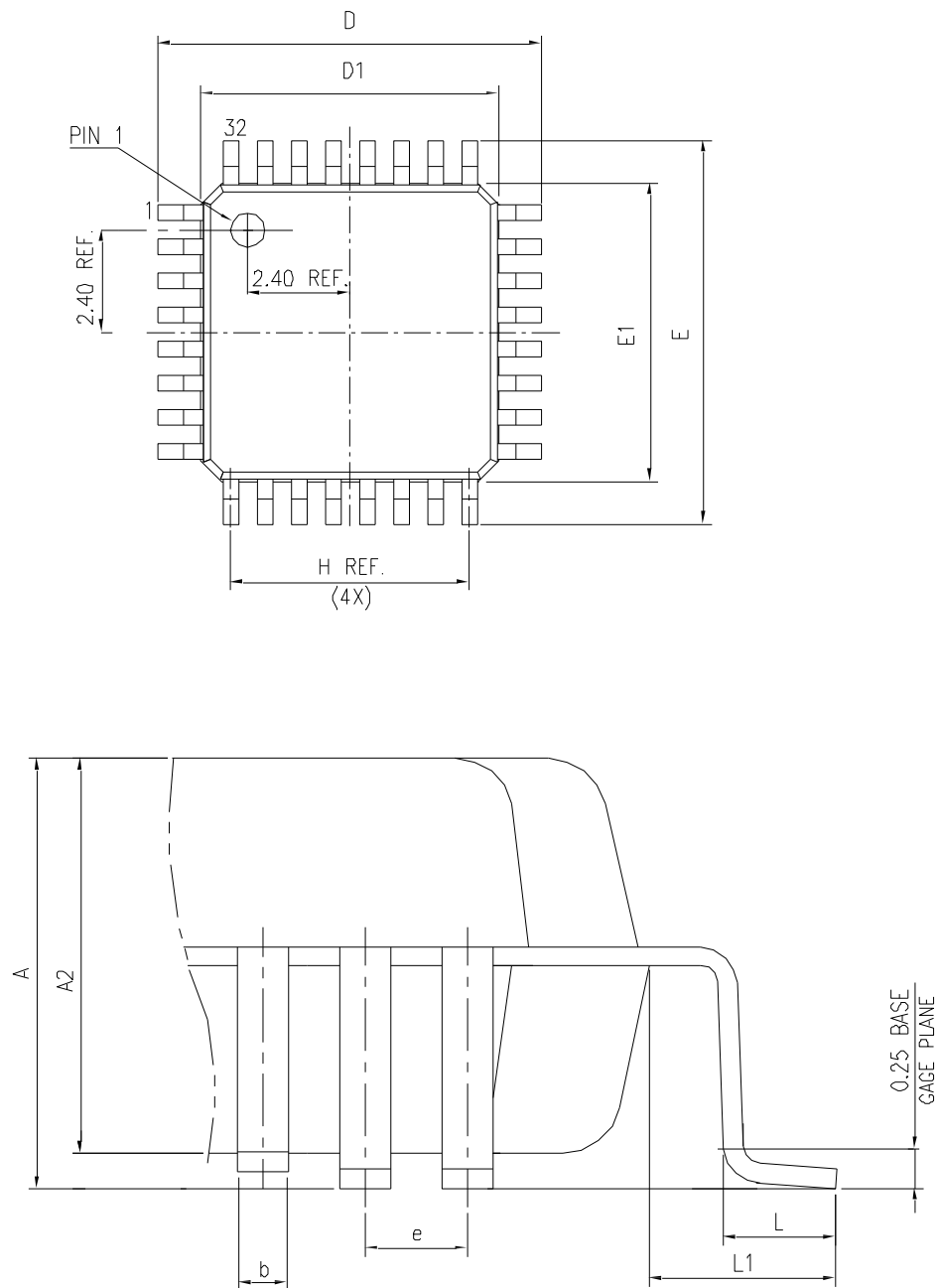
图23 LQFP32 封装图
