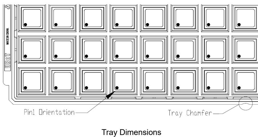
图33 托盘包装示意图
