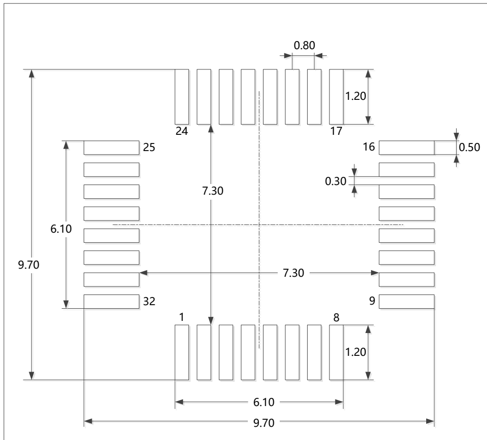
图24 LQFP32 焊接 Layout 建议
