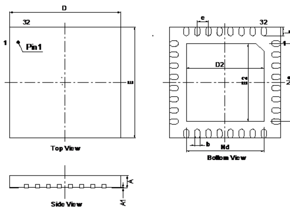
图29 QFN32 封装图
