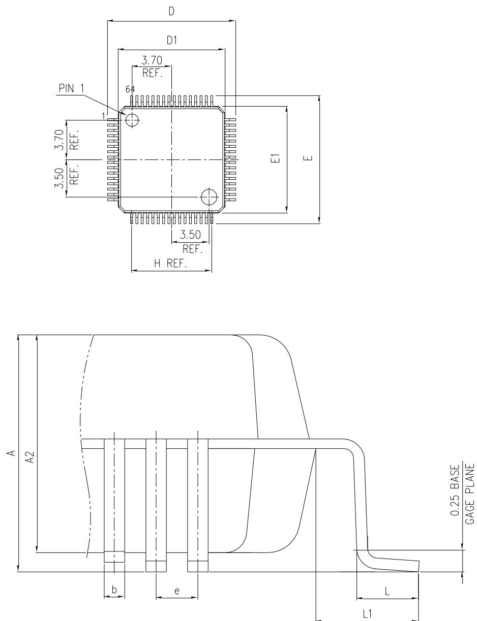
图17 LQFP64 封装图
