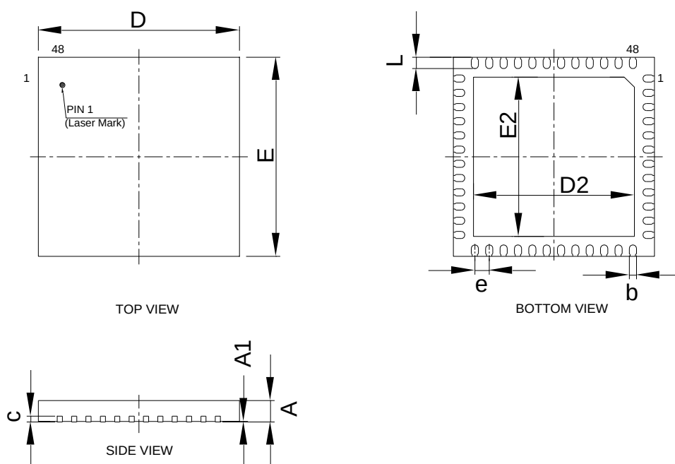
图 25 QFN48 封装图
