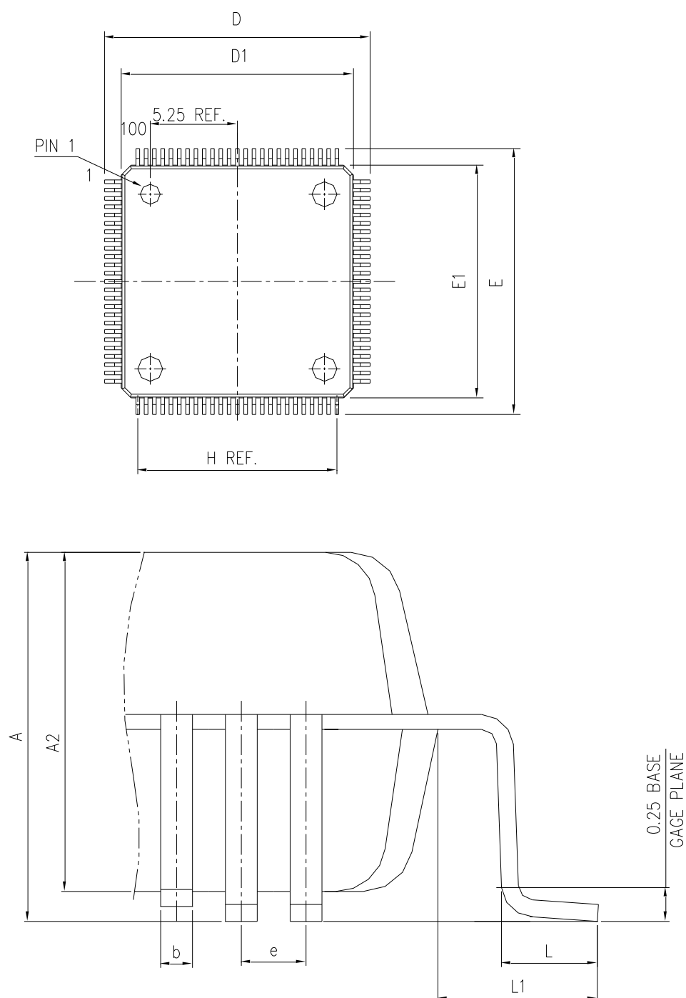
图 16 LQFP100 封装图
