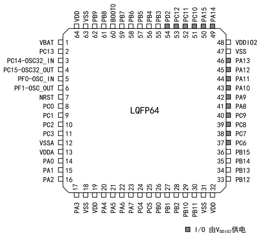
图 2 APM32F072xBT7 系列 LQFP64 引脚分布图
