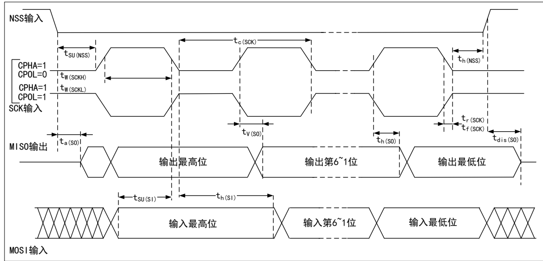
图 13 SPI 时序图—从模式和 CPHA=1
