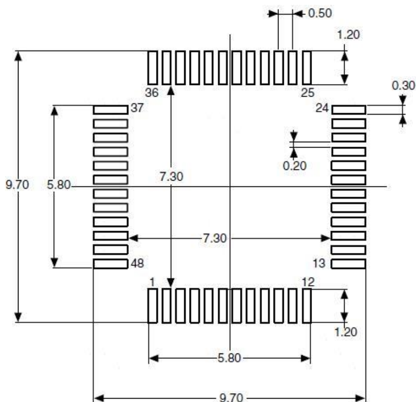
图 19 LQFP48 焊接 Layout 建议
