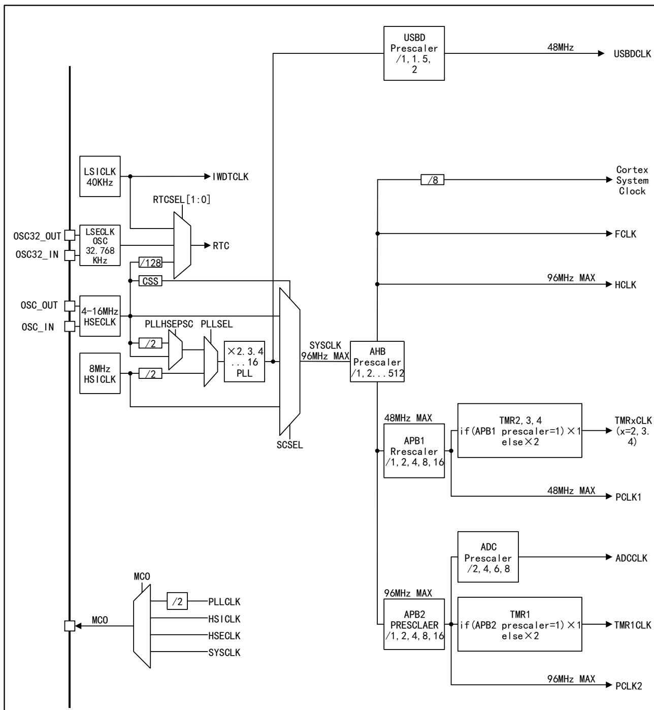
图 5 APM32F103x4x6x8 时钟树
