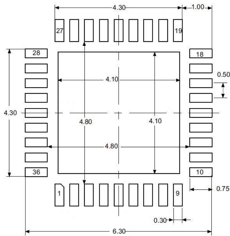
图 22 QFN36 焊接 Layout 建议
