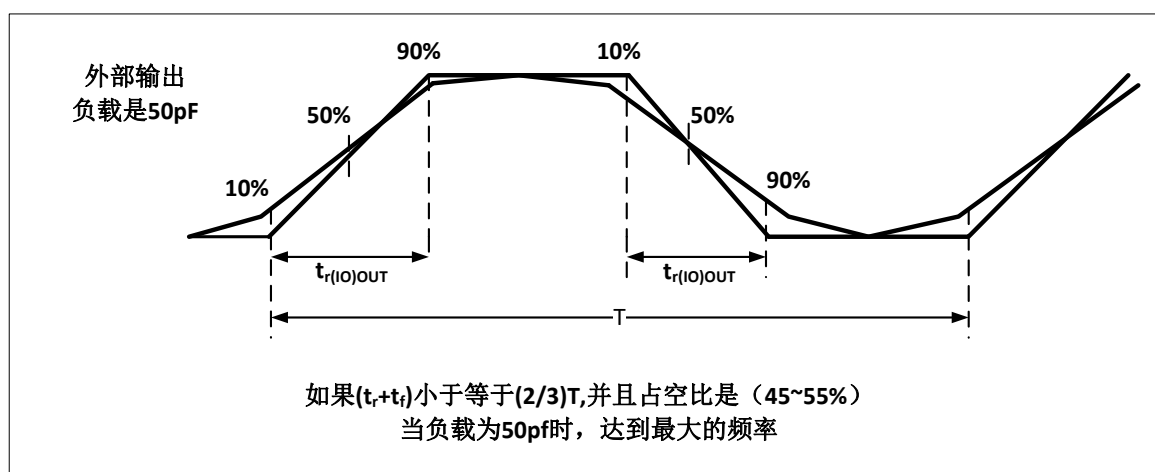
图 10 输入输出交流特性定义
