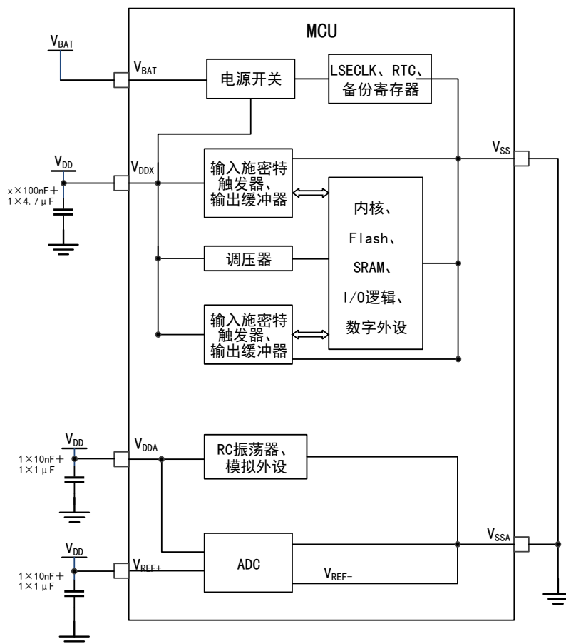
图 6 电源方案
