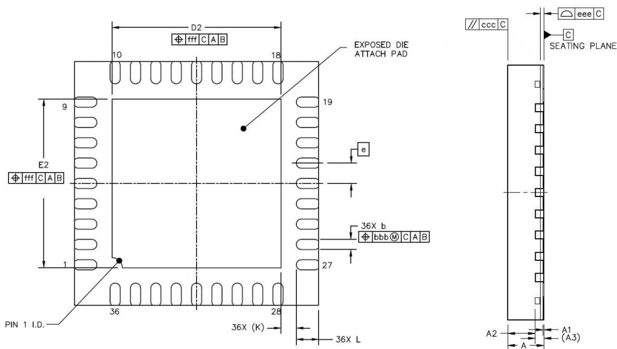
图 21 QFN36 封装图
