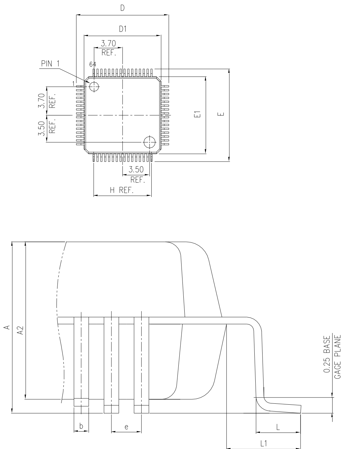
图 15 LQFP64 封装图
