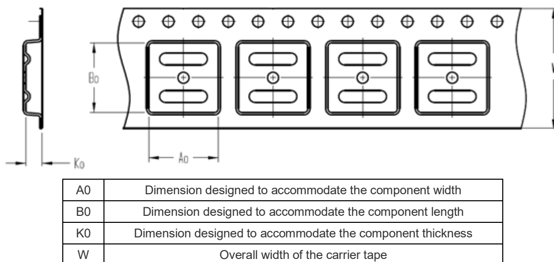
图 24 带状包装规格图
