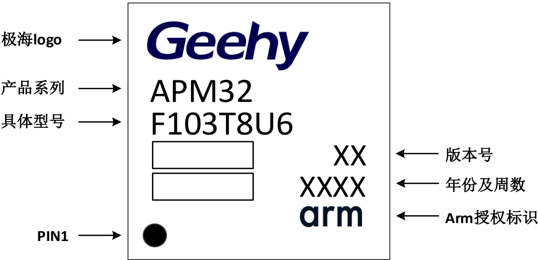
图 23 QFN36 标识图
