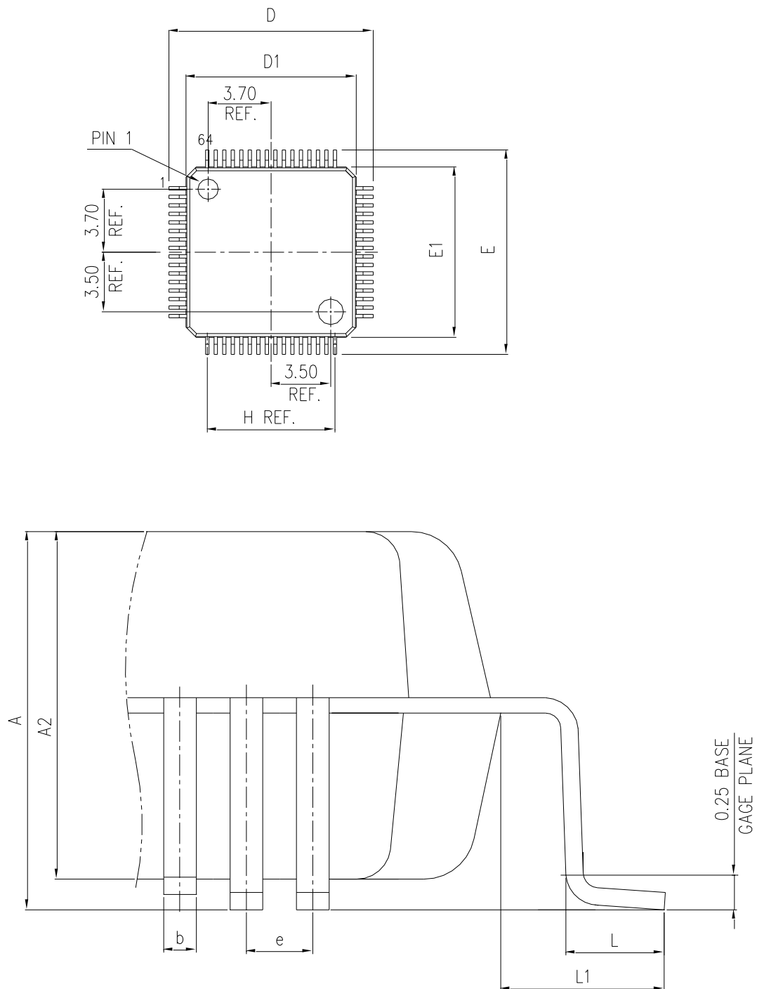
图23 LQFP64 封装图
