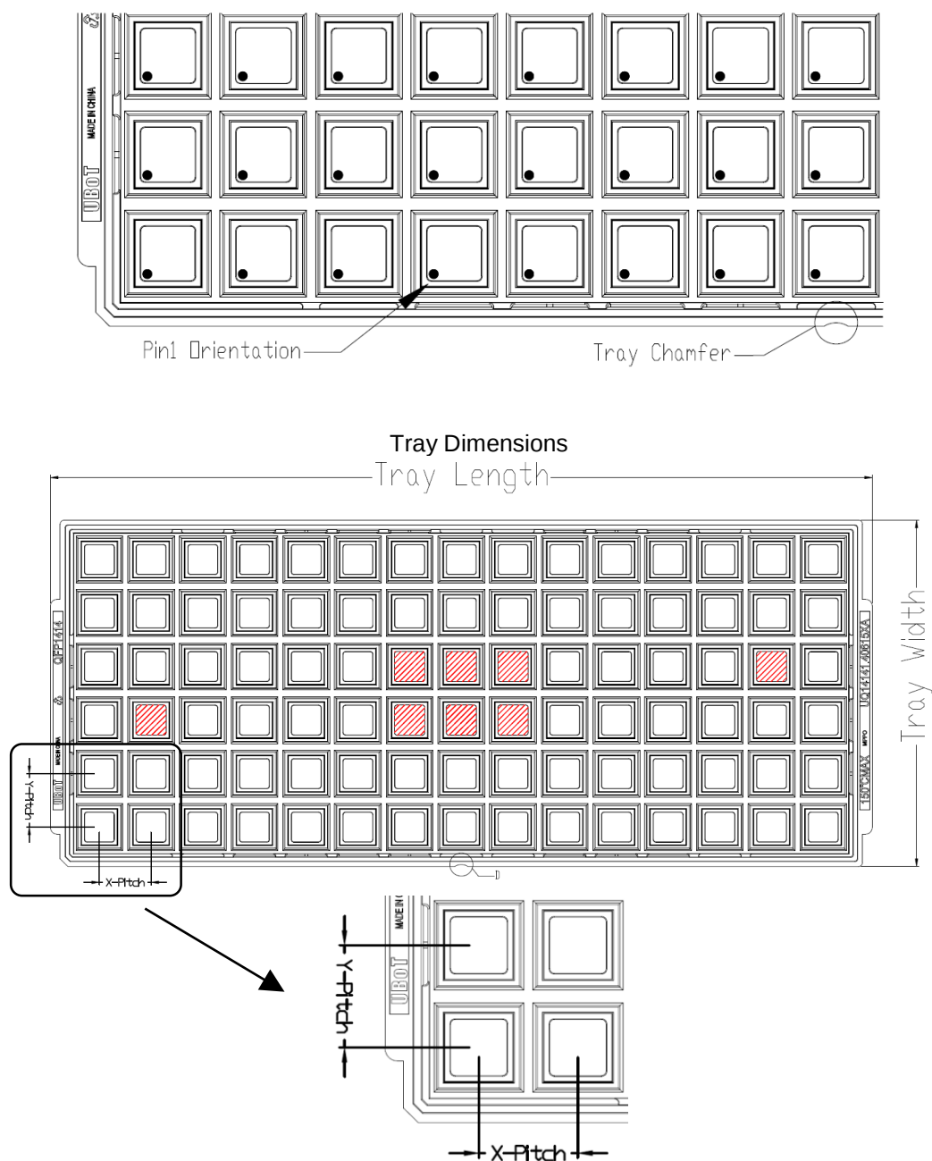
图27 托盘包装示意图
