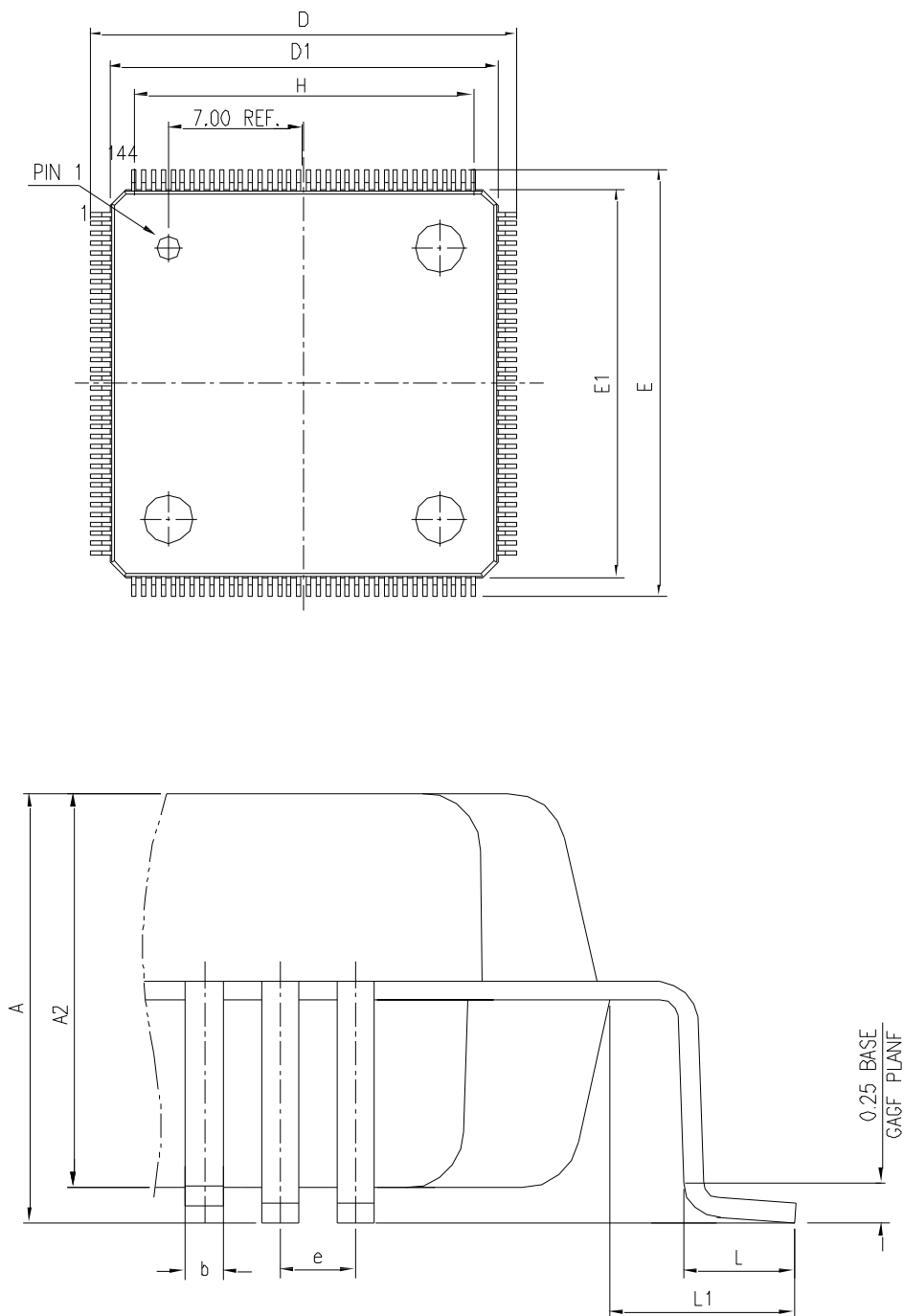
图17 LQFP144 封装图
