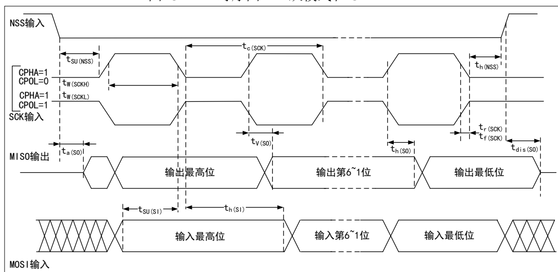
图13 SPI 时序图 — 从模式和 CPHA=1 (1)
