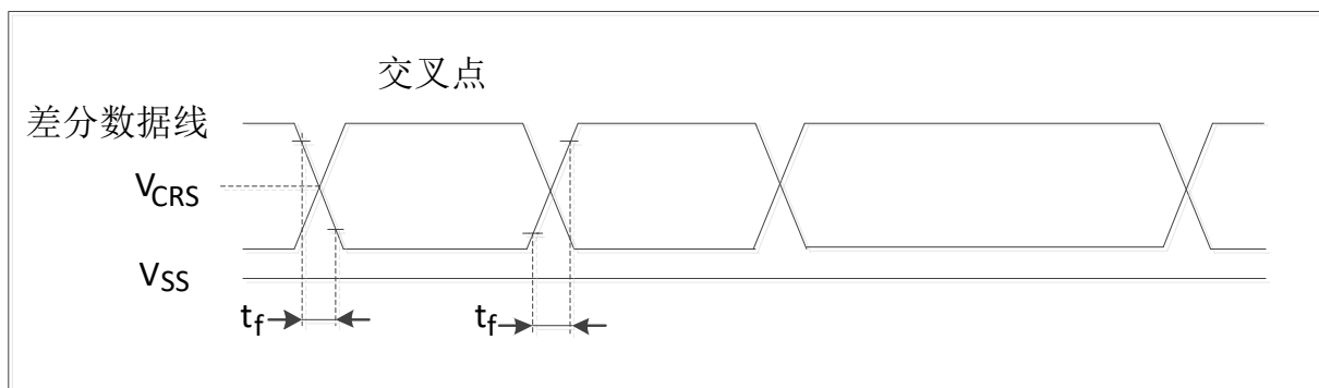
图15 USB2 时序：数据信号上升和下降的时间定义
