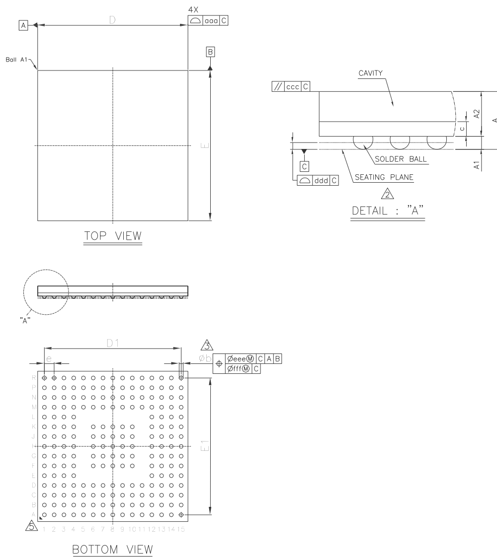
图 29 BGA176+25 封装图
