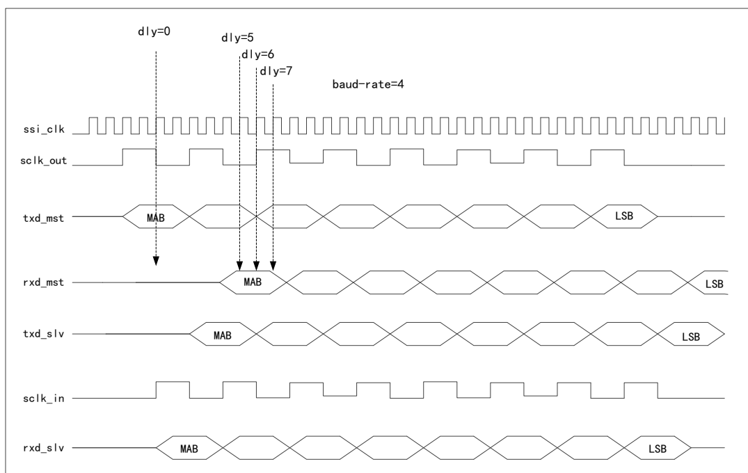
图 96 利用 QSPI 采集 RXD 信号样品
