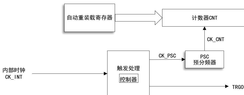
图 61 基本定时器结构框图
