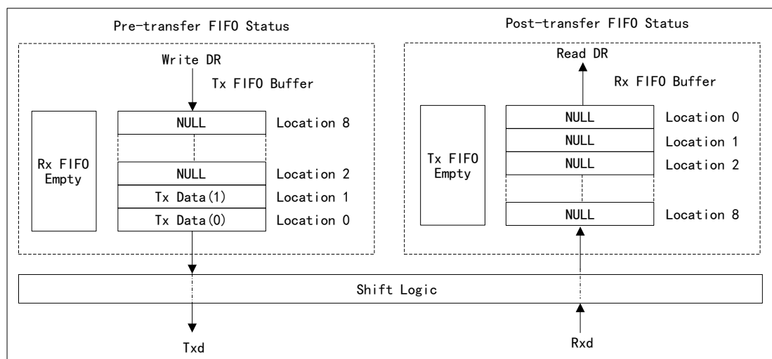
图 91 发送状态下的 QSPI 传送 FIFO 状态
