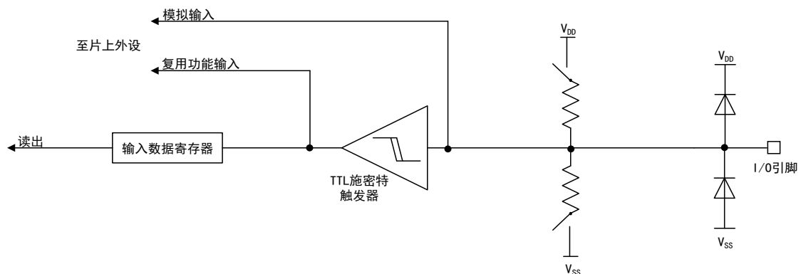
图 14 输入模式结构
