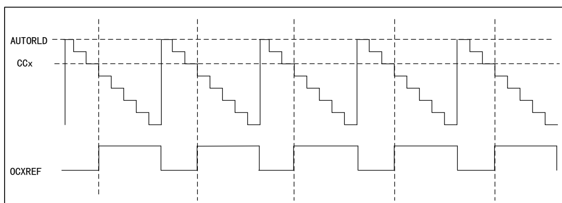
图 23 PWM1 向下计数模式的时序图
