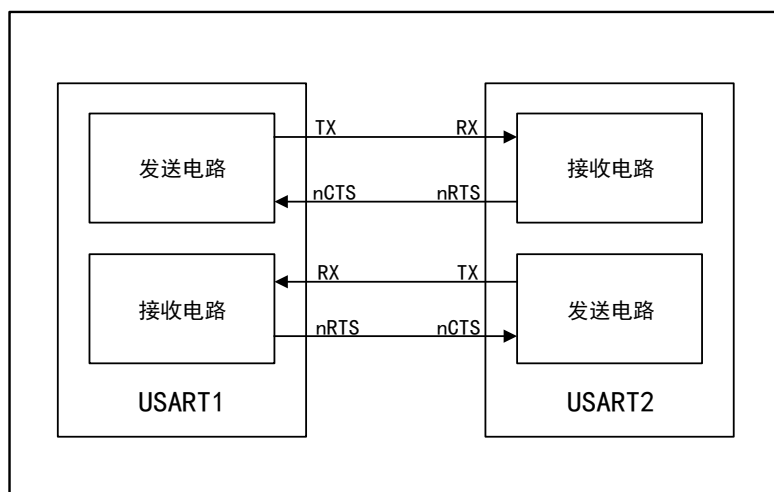
图 76 两个 USART 之间的硬件流控制
