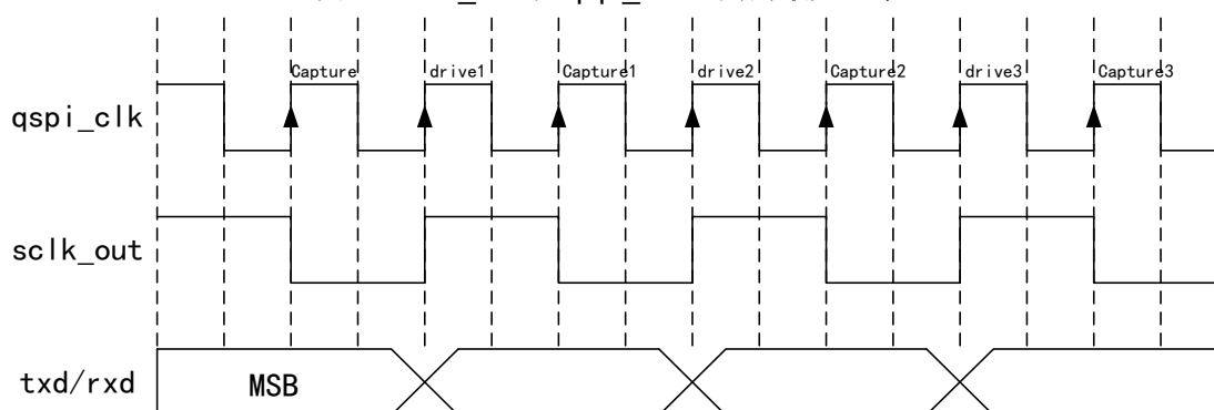
图 94 sclk_out 和 qspi_clk 之间的最大比率
