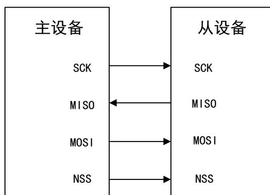
图 86 全双工模式连接
