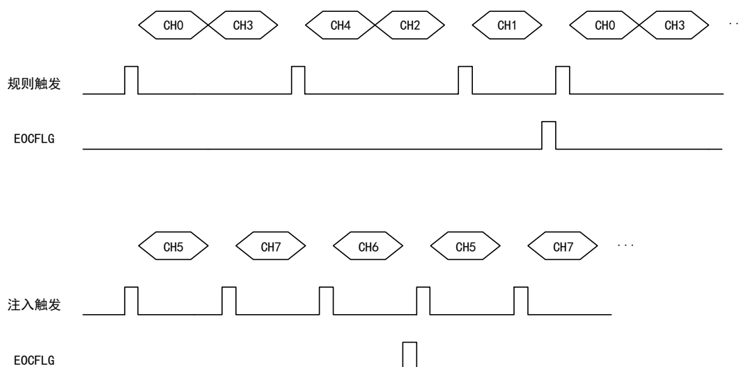
图 117 间断模式时序图
