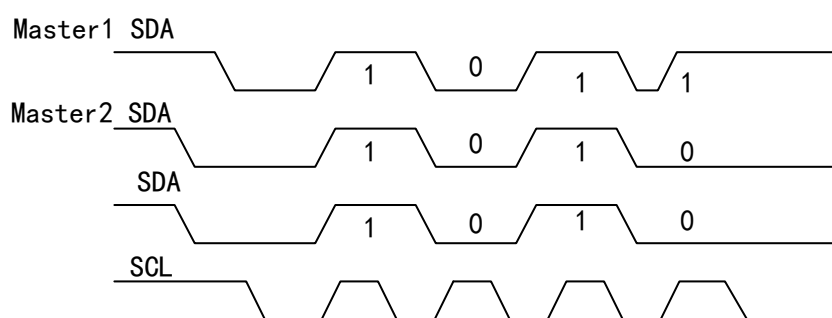
图 85 SDA 时序图
