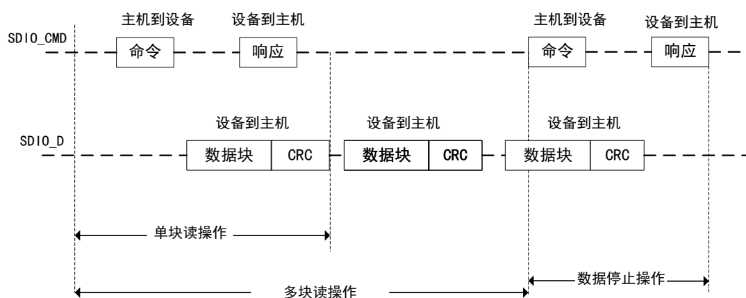
图 108 SDIO（多）数据块读操作
