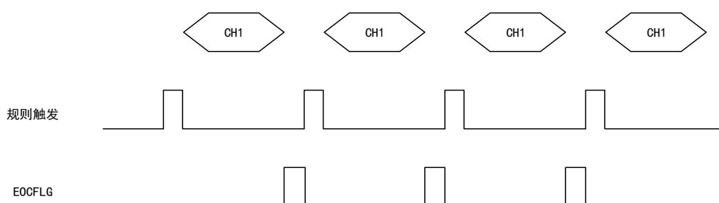
图 114 单次转换模式时序图
