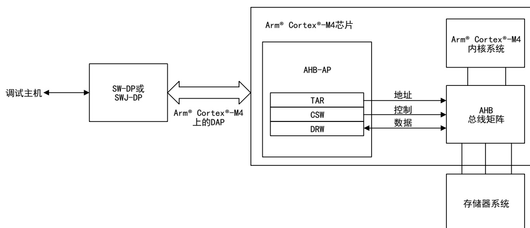
图 12 APM32F425xG_F427xG 级别和 Arm® Cortex®-M4F 级别的调试框图
