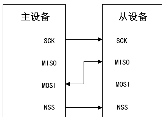
图 89 双向线连接
