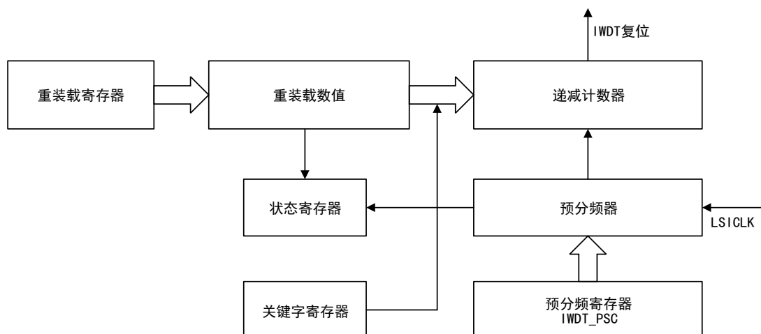
图 63 独立看门狗结构框图
