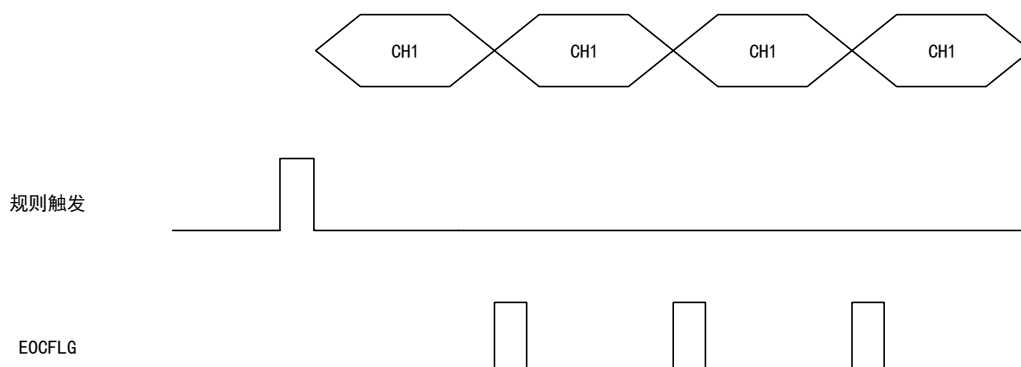
图 115 连续转换模式时序图
