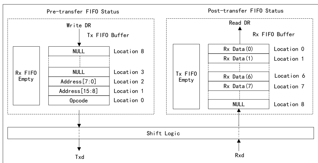
图 93 EEPROM 读取传输模式下的 FIFO 状态
