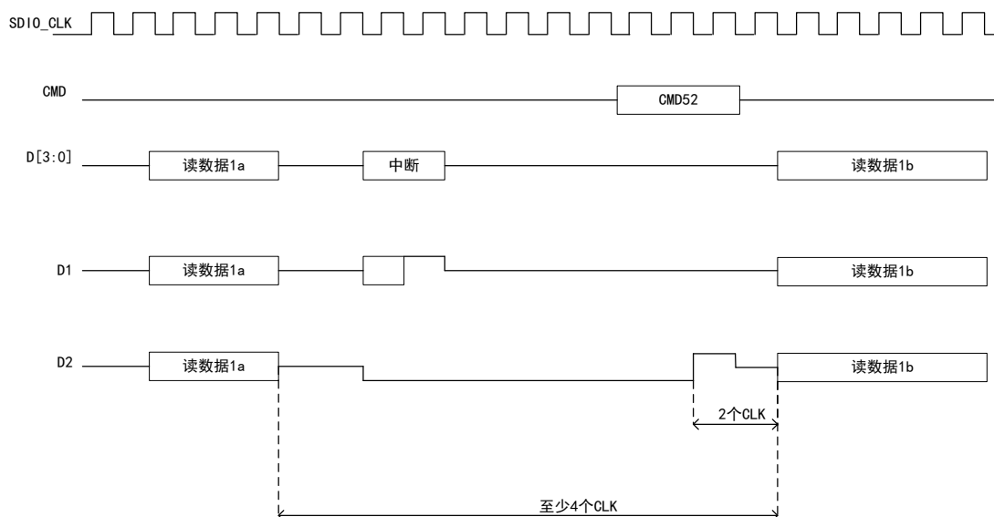
图 112 使用 SDIO_D2 信号线的读等待操作
