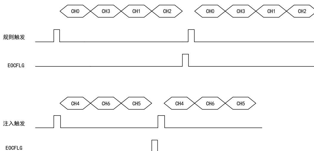
图 116 扫描模式时序图
