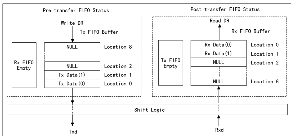
图 90 发送和接收状态下的 QSPI 传送 FIFO 状态
