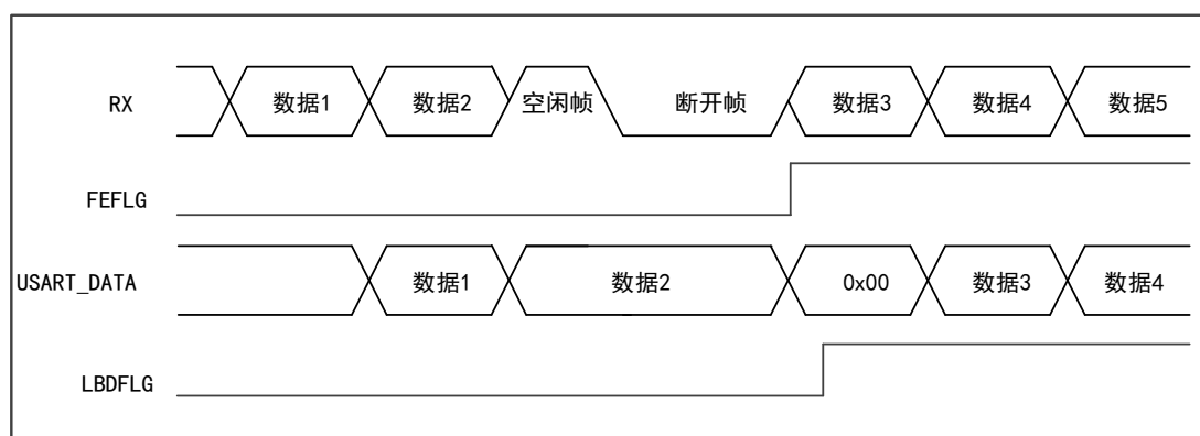
图 72 空闲状态检测断开帧
