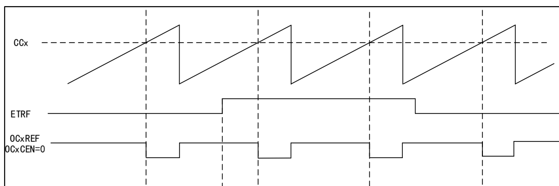
图 36 OCxREF 时序图
