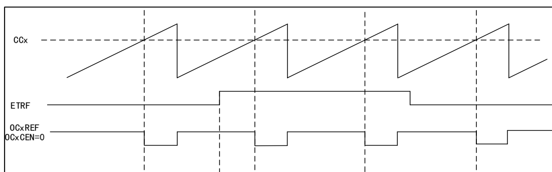
图 52 OCxREF 时序图
