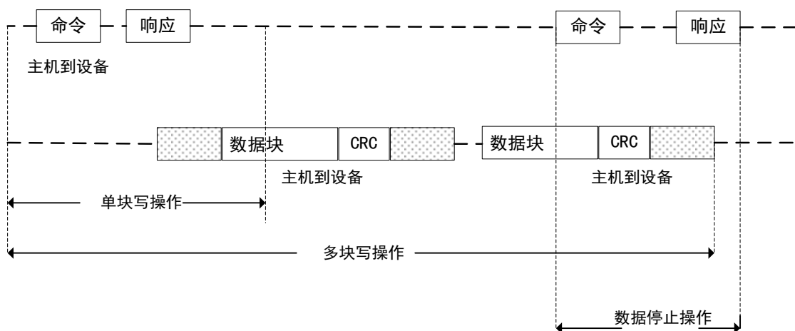
图 109 SDIO（多）数据块写操作
