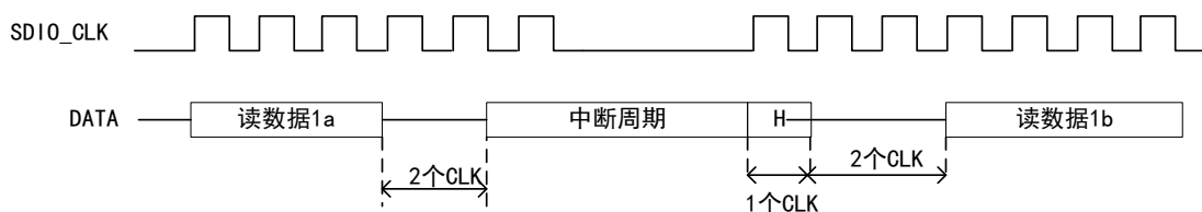
图 113 通过停止 SDIO_CLK 的读等待操作
