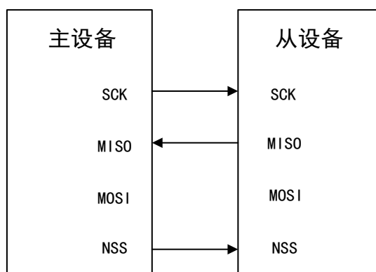
图 87 半双工模式连接（主机用来接收，从机用来发送）
