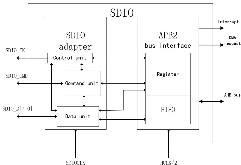
图 106 SDIO 结构框图
