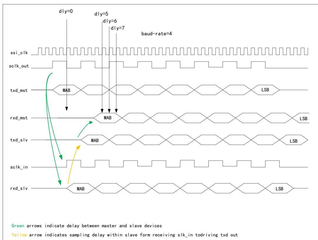
图 95 接受数据（RXD）样本延迟描述
