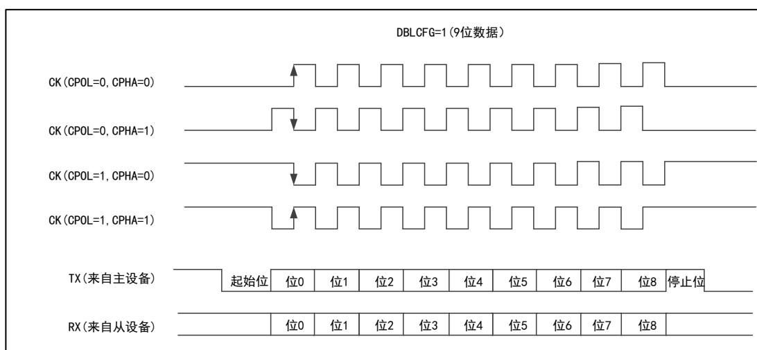
图 71 USART 同步发送时序图 (DBLCFG=1)
