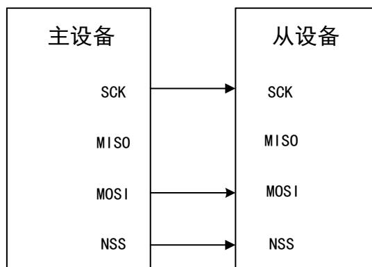
图 88 半双工模式连接（主机只发送，从机接收）
