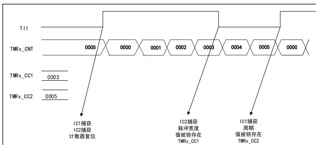
图 57 PWM 输入模式时序图
