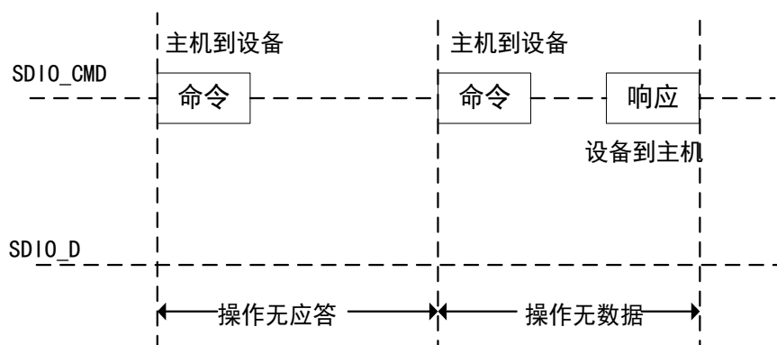
图 107 SDIO “无响应”和“无数据”操作
