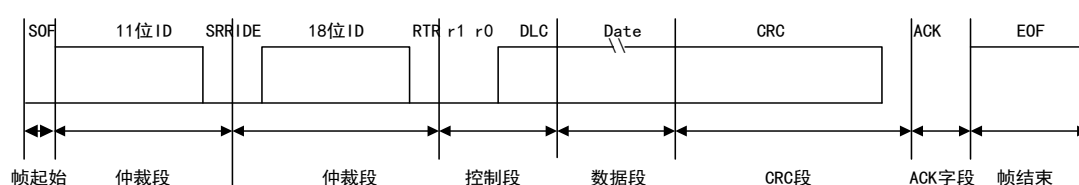
图 98 扩展数据帧
