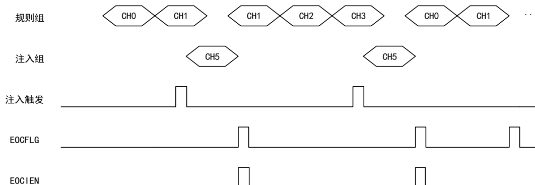
图 118 触发注入时序图
