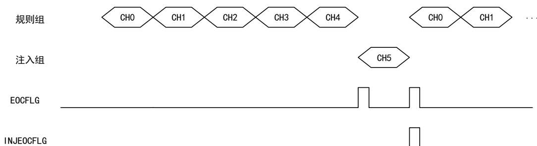
图 119 自动注入时序图
