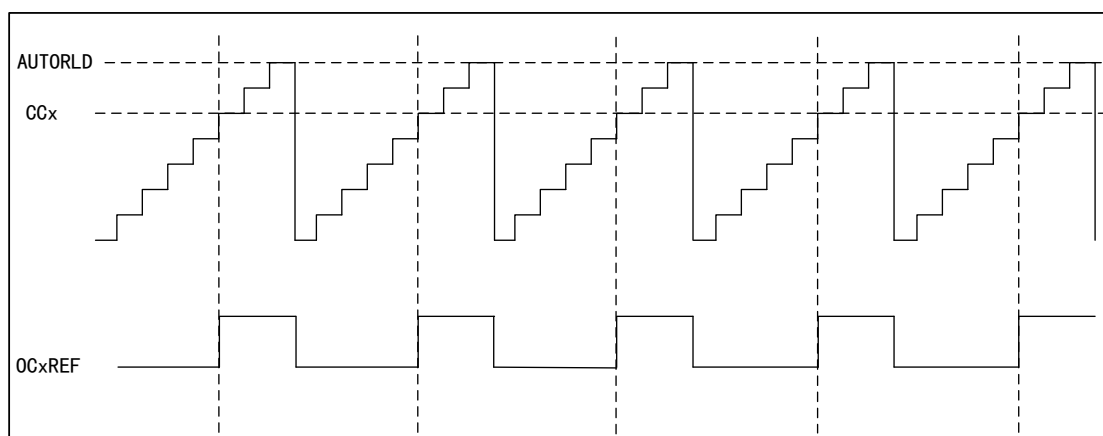
图 45 PWM2 向上计数模式的时序图
