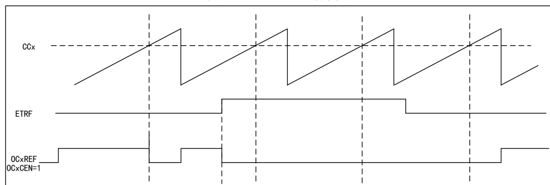
图 37 OCxREF 时序图
