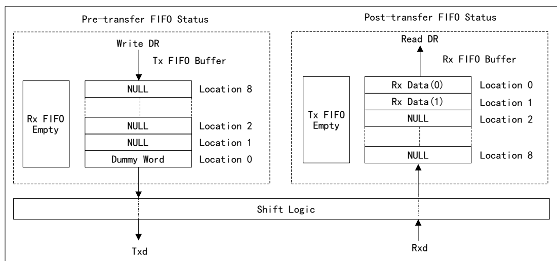
图 92 仅接收状态下的 QSPI 传送 FIFO 状态
