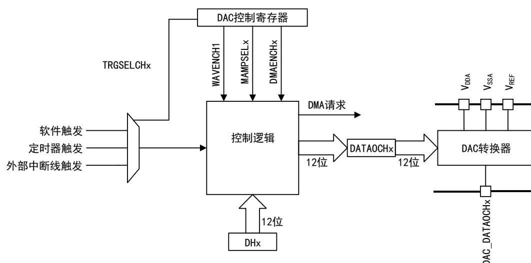
图 121 DAC 结构框图
