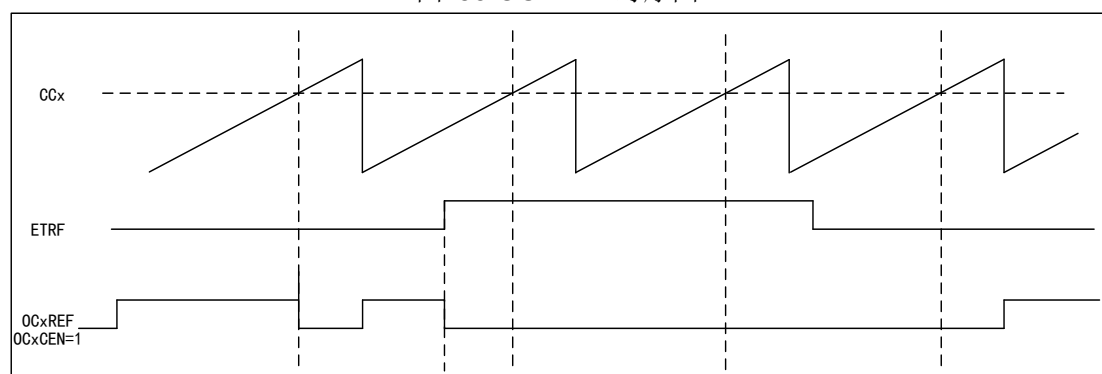
图 53 OCxREF 时序图
