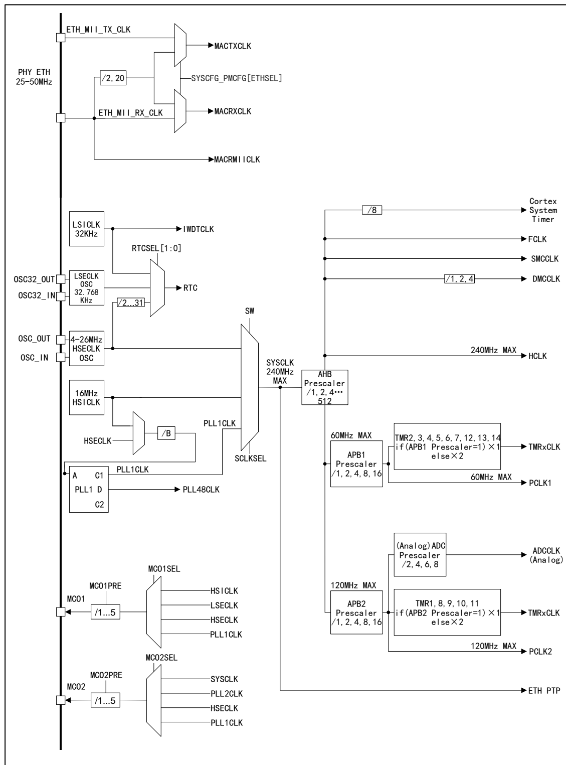
图 6 APM32F425xG_F427xG 时钟树
