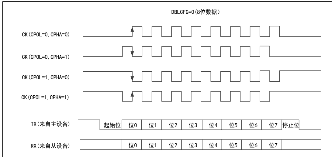
图 70 USART 同步发送时序图 (DBLCFG=0)
