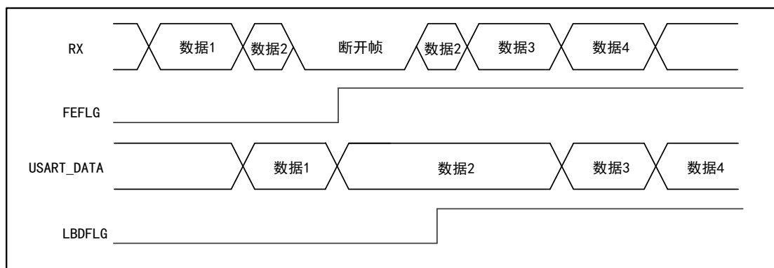
图 73 数据发送状态检测断开帧
