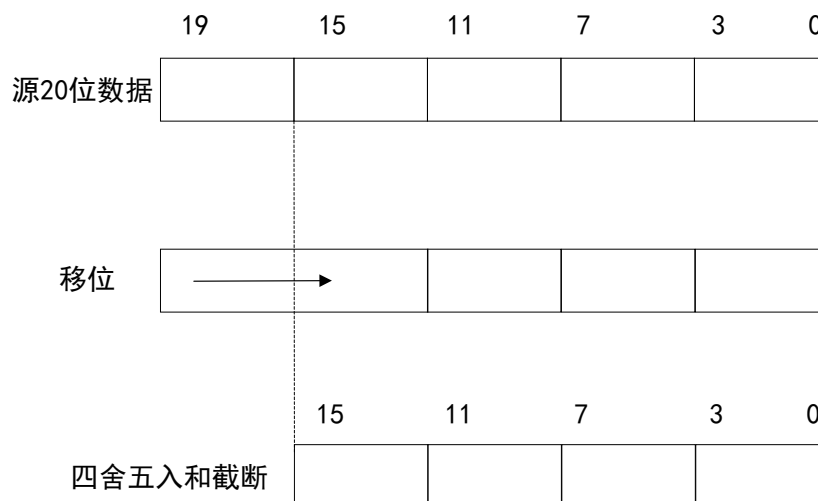
图 120 20 位到 16 位的结果截断
