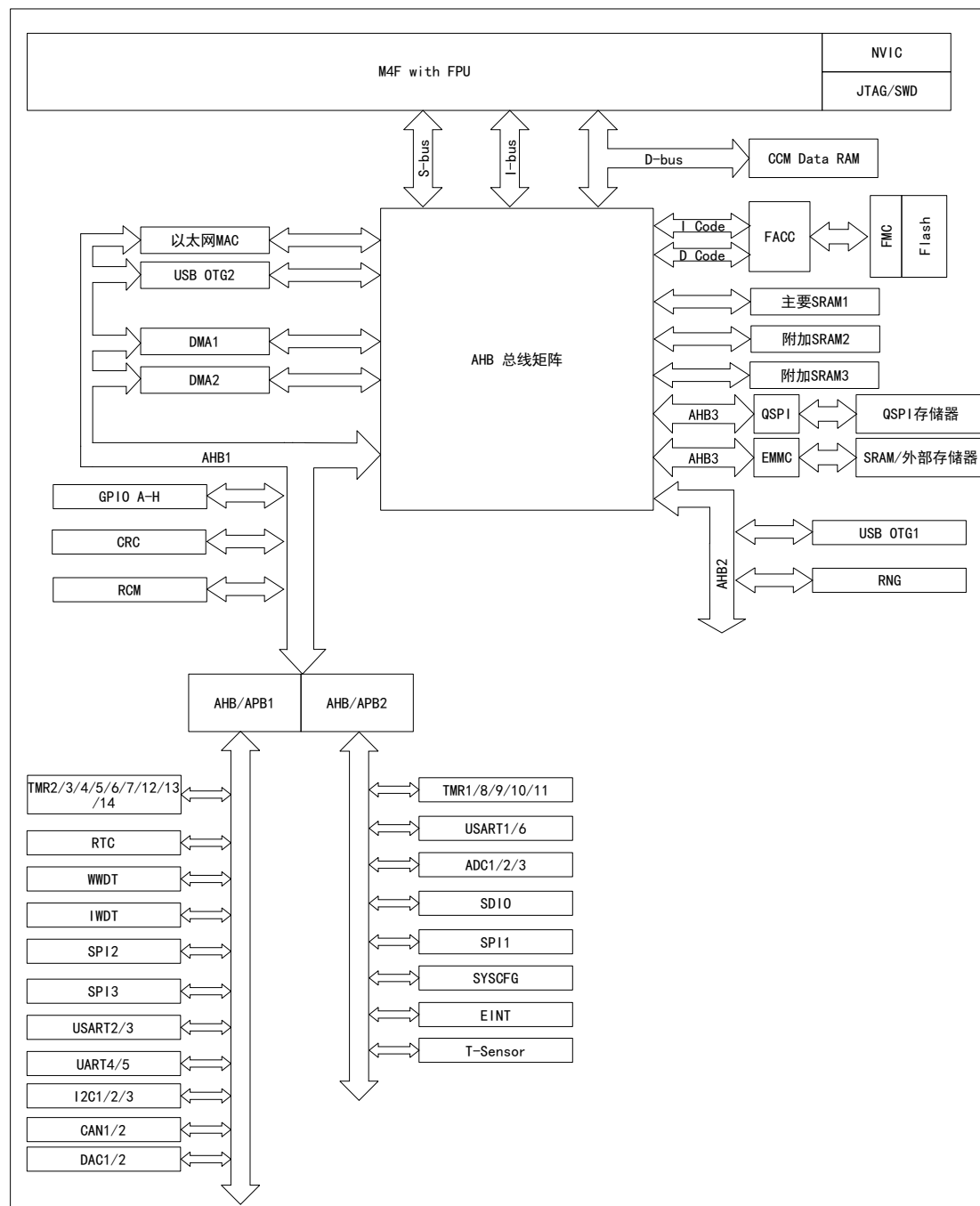
图 1 APM32F425xG_F427xG 系统架构框图
